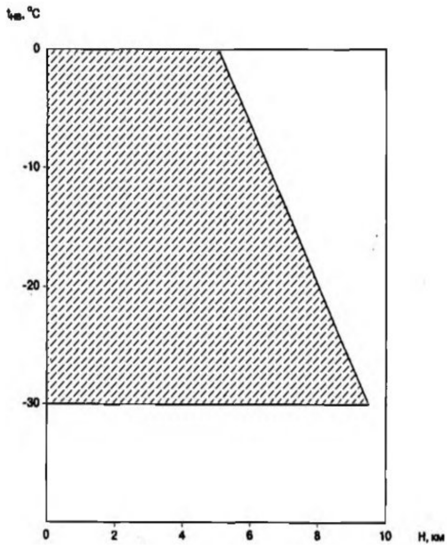
Рисунок Е3. Зона возможного обледенения, определяемая высотой и температурой наружного воздуха, для условий максимального длительного обледенения
