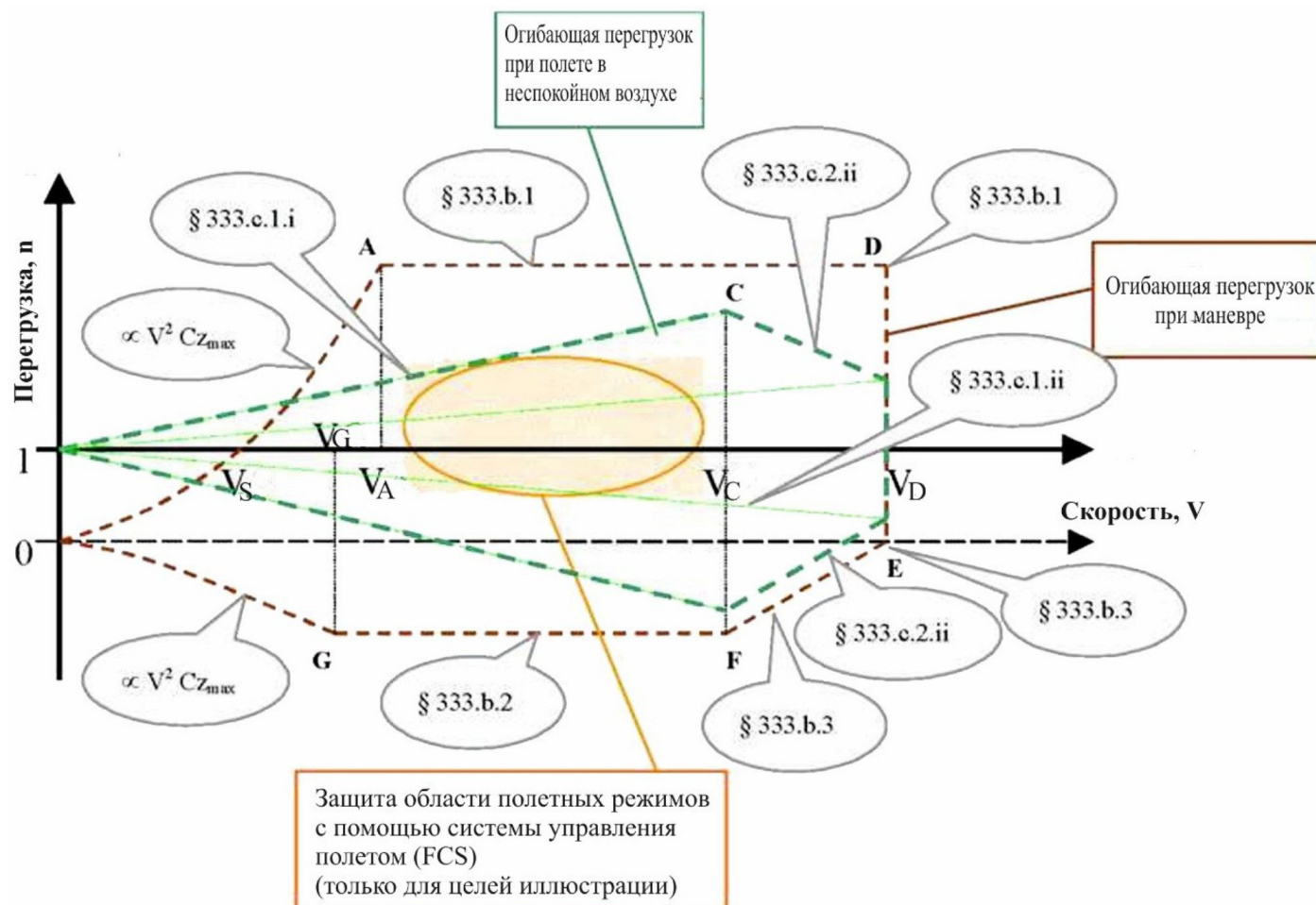
Рисунок С1. Область полетных режимов
