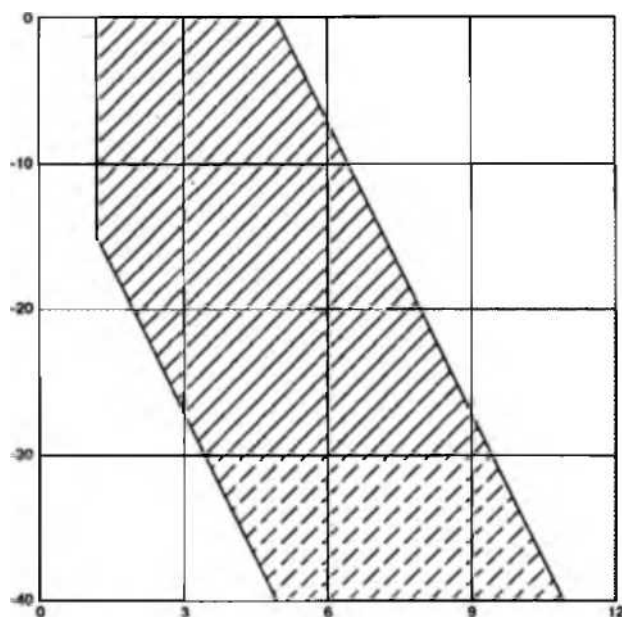
Рисунок Е5. Зона возможного обледенения, определяемая высотой и температурой наружного воздуха, для условий максимального кратковременного обледенения.
