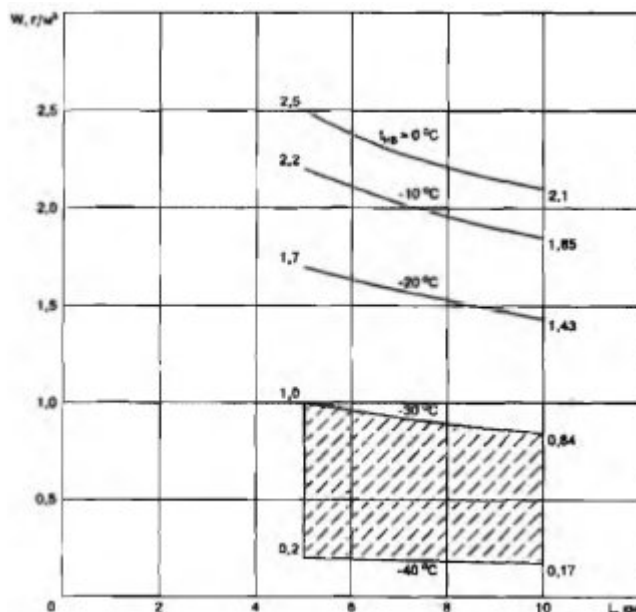
Рисунок Е4. Зависимость водности от горизонтальной протяженности зоны обледенения в условиях максимального кратковременного обледенения в диапазоне высот от 1200 до 11000 м для облаков (кучевообразных) со среднеарифметическим диаметром капель 20 мкм.
