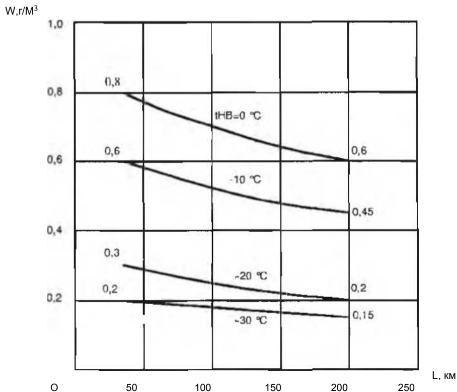
Рисунок Е1. Зависимость водности от горизонтальной протяженности зоны обледенения в условиях максимального длительного обледенения в диапазоне высот от 0 до 9500 м для облаков (слоистообразных) с максимальной вертикальной протяженностью 2000 м. и среднеарифметическим диаметром капель 20 мкм.
